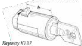
Keyway K137
