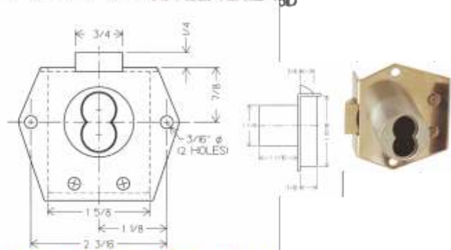
IC Rim Latch Right Hand Door OL725RL/DR-DM-26D
